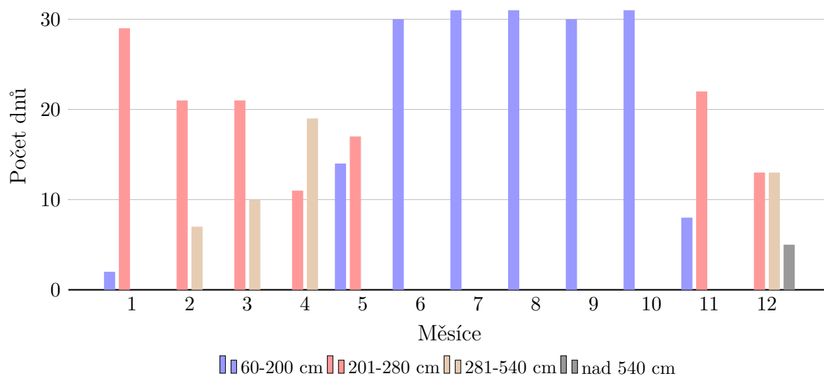
Setrvalost vodních stavů v regulovaném úseku dolního Labe v roce 2023
